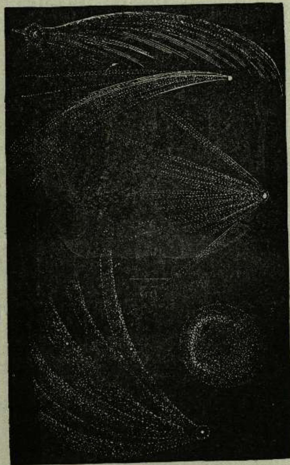
KOMETOS.
