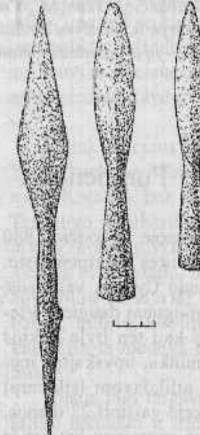
Pav. 4. Ietigaliai iš Norelių kapinyno
