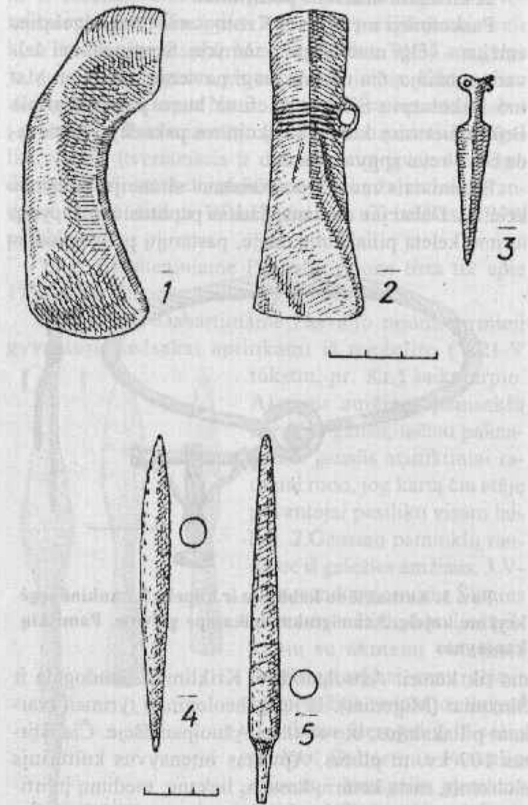
Pav. 2. Akmens ir žalvario amžiaus radiniai. 1-2 Vaškų lobis: 1. Haličo tipo pentinis kirvis, 2. Melaro tipo įmovinis kirvis, 3. Durklas. 4-5. Raginiai šėivos pavidalo strėlių antgaliai
